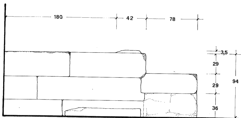
Prospetto AA'
